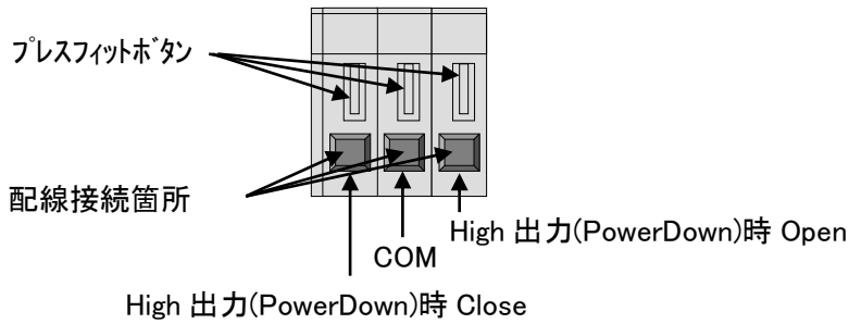
図 接点出力ピン配置
